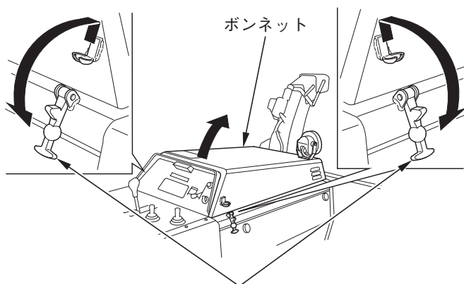
ボンネット キャッチ
